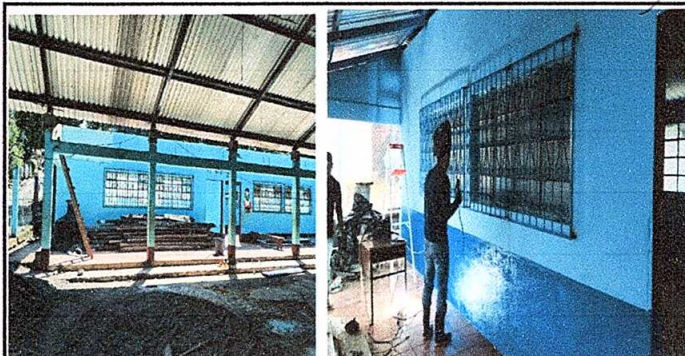
Foto No. 4: En proceso de la aplicación de pintura en muros exteriores e interiores.
