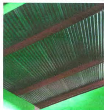
Foto 4: Reparación de sistema eléctrico: Sustitución de focos ahorradores, flaponeras, interruptores, toma corrientes, flipones, cableado eléctrico, ducto eléctrico + accesorios.
