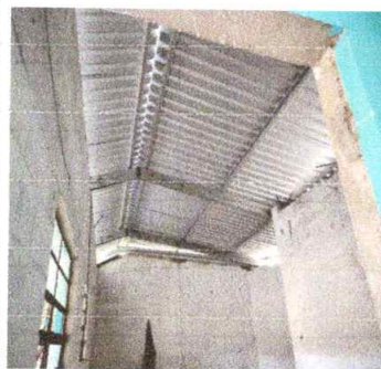
Foto 3: Sustitución de estructura de soporte de madera por metal
