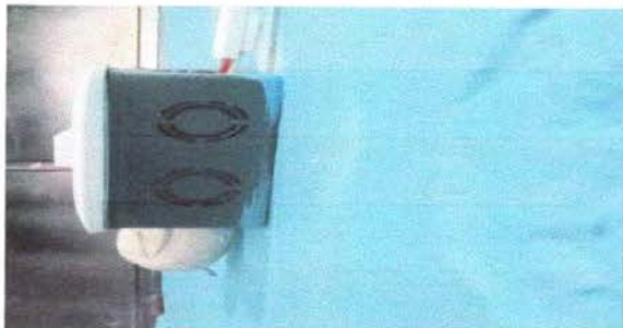
FOTO 16: Sustitución de cajas octagonales
