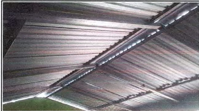
Sustitución de lámina por lámina troquelada aluzinc calibre 26 de 12 pies
