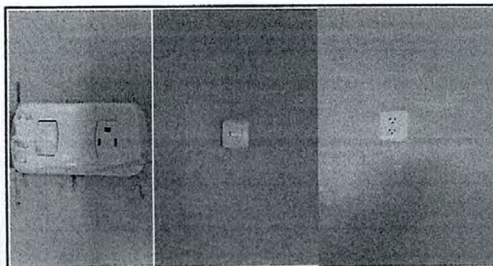
Foto 11: Sustitución de toma Corriente y Apagadores
