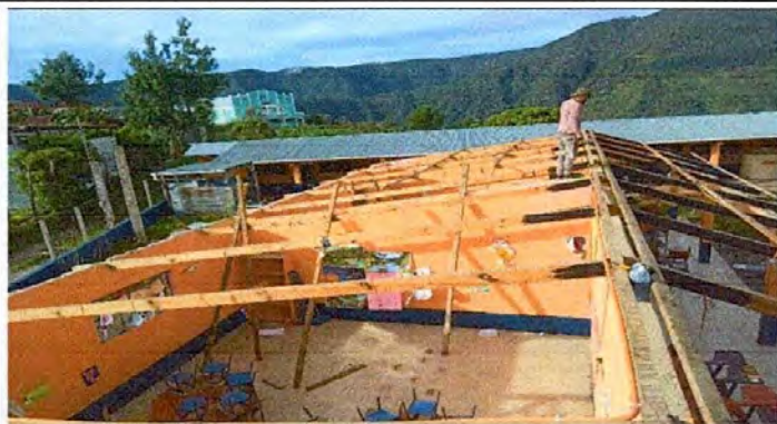
Foto1: Sustitución de lamina de cocina por lámina troquelada
