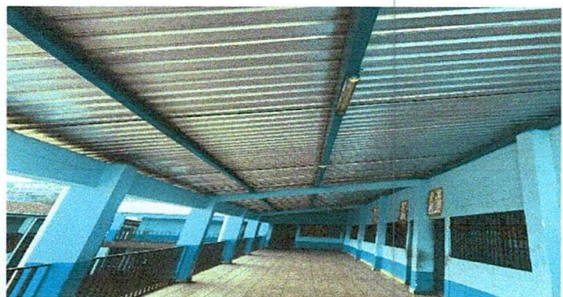
Foto 5: Techo aulas 1, 2 y 3
