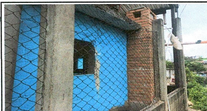
Foto 5: Sustitución de chimenea de tubo de concreto por ladrillo
