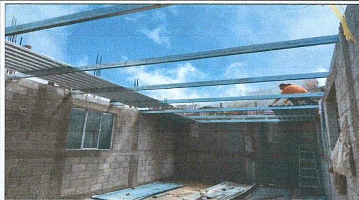
Foto 1: colocando las vigas y las laminas en el techo del aula
