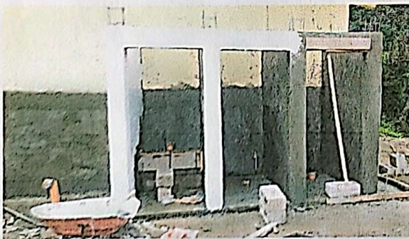
Foto 5: Los baños necesitaron repello, colocación de inodoros lavables y mingitorio, instalación de techo a base de estructura de metal y sustitución de torta de cemento por azulejo en el piso.
