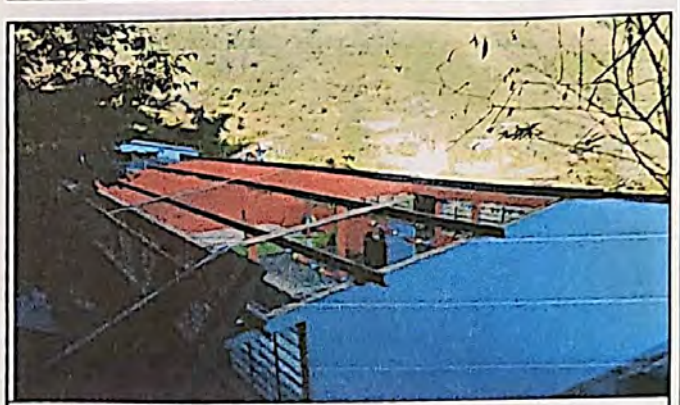
Foto 4: Pintura de costaneras de dos aulas
