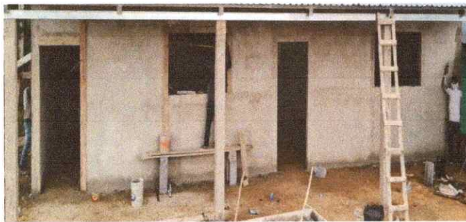
FOTO 3: SUSTITUCIÓN DE VENTANAS DE MADERA POR METAL
