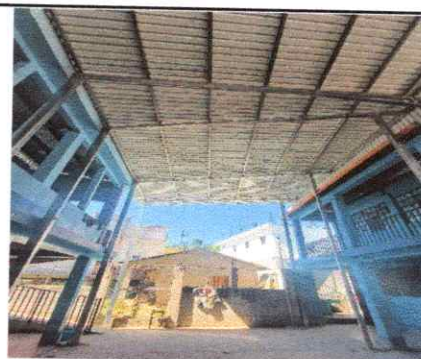
Foto 6: estructura de soporte de metal y techado de lmina troquelada
