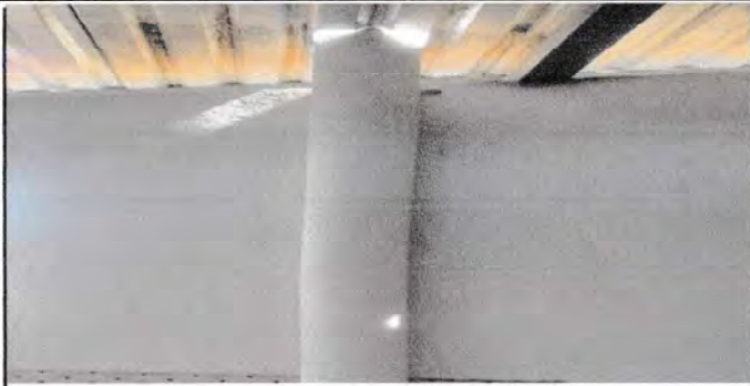
Foto 1: REPARACIÓN DE REPELLO Y CERNIDO EN PAREDES EN MODULO DE COCINA DE PRIMARIA DE ALDEA EL GRANADILLO
