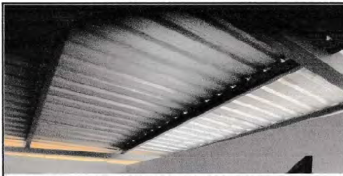
Foto 3: SUSTITUCIÓN DE LAMINA TROQUELADA EN MODULO DE PRIMARIA DE ALDEA EL GRANADILLO
