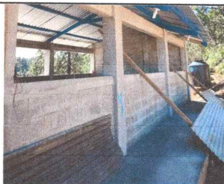
Foto 4: Sustrucción de ventanas de madera de metal mas vidrio 320 x 110
