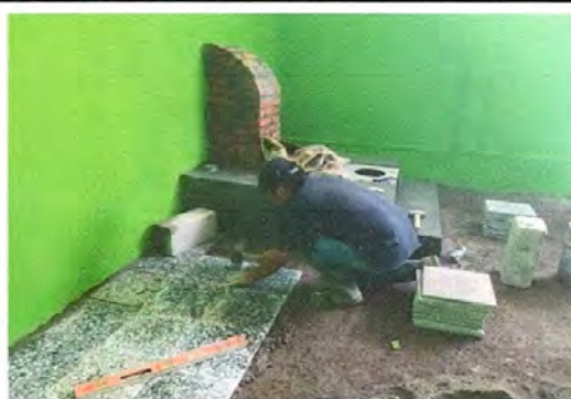
Foto 4: Se esta colocanco el piso de granito en la cocina.
