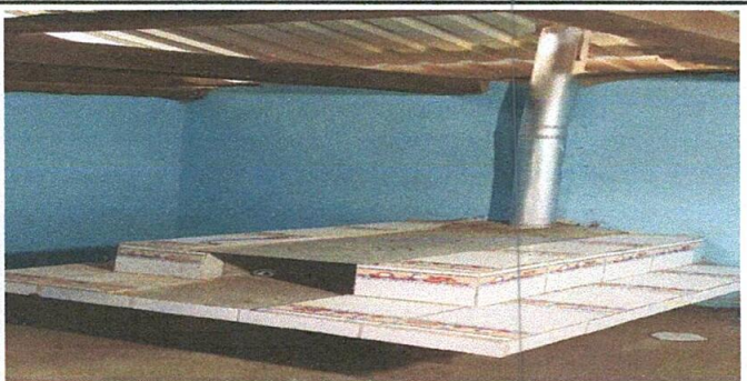
Mejoramiento de cocina finalizado
