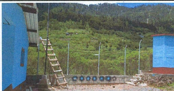
FOTO 5: REPARACIÓN DE MURO PERIMENTAL CON TUBO HG Y MALLA
