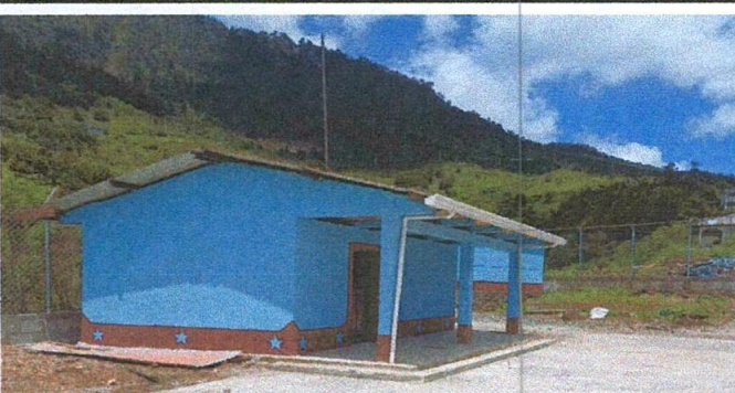
FOTO 3: REPARACIÓN DE REPELLO Y CERNIDO DE PAREDES
