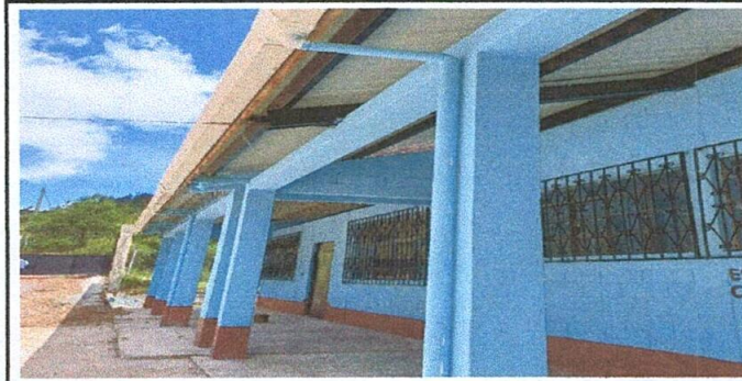
FOTO 6: CANALES Y BAJADA DE AGUA PLUVIAL
