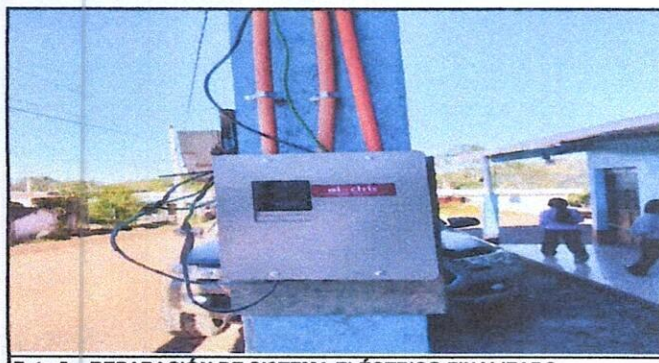
Foto 5: REPARACIÓN DE SISTEMA ELÉCTRICO FINALIZADO
