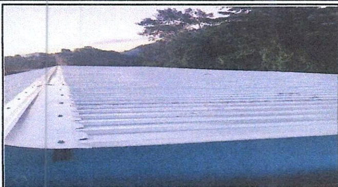
Foto1: SUSTITUCIÓN DE LÁMINA, POR LÁMINA TROQUELADA ALUZINC CALIBRE 26 FINALIZADO
