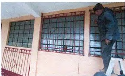
foto 17: sustitución de balcones de metal color rojo óxido 1.76 m x 1.31 m, 2.02 m x 1.31 m, 1.01 m x 1.31 m, 1.75 m x 1.31 m, 1.98 m x 1.31 m, 1.80 m x 1.35 m, 2.02 m x 1.35 m, 1.79 m x 1.35 m, 2.05 m x 1.35 m
