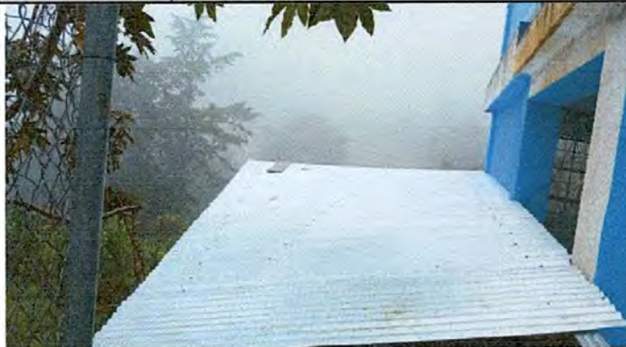
Foto 7: Sustrucción de techo de baños: láminas acanaladas y vigas de madera por estructura metálica (costaneras) con láminas acanaladas calibre 26
