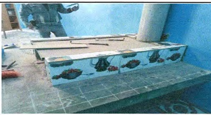
Foto 12: Sustitución de chimenea de concreto
