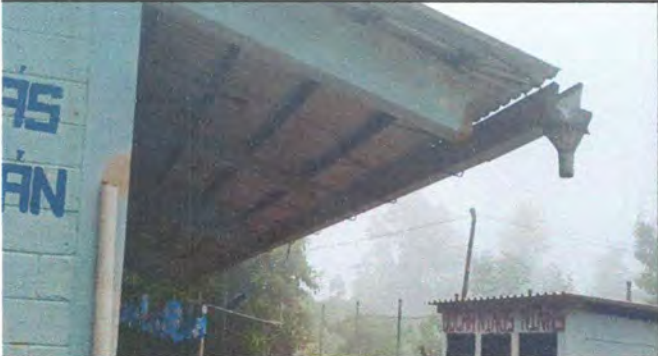
FOTO 3: Los canales están quebrados y los conos para recibir el agua están oxidados y otros ya se arruinaron completamente.
