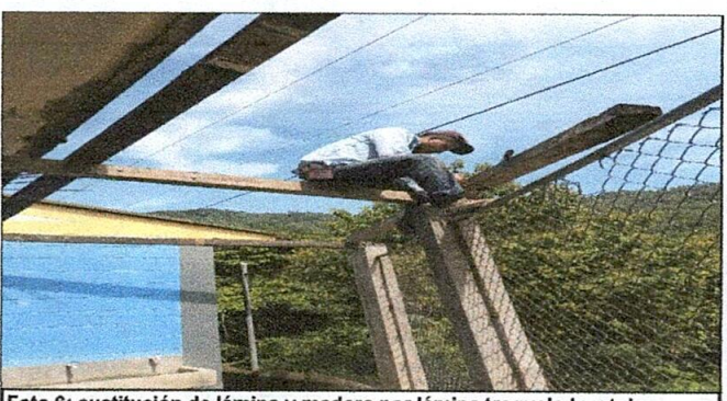
Foto 6: Sustrucción de lámina y madera por lámina troquelada y tubo galvanizado
