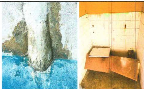
Foto 4: Sustrucción de tubería pvc línea principal de aguas negras
