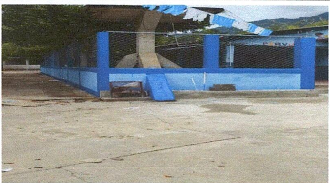
Foto 5: MURO PERIMETRAL: reparación de muro de block con malla galvanizada, soleras intermedias y columnas.
