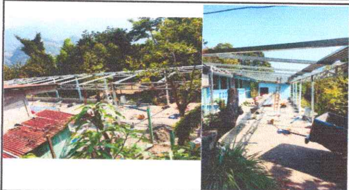
Foto1: Sustitución de lámina, por lámina troquelada aluzinc calibre 26-168 mts. Cuadrados.
