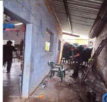
Foto 16: Sustitución de estructura de metal de ventana
