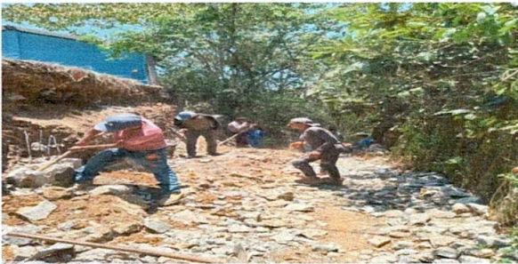
Foto 5: Muro de Contención (durante)
