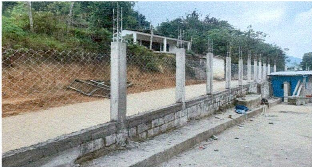
Foto 3: Columnas de muro perimetral (despues)
