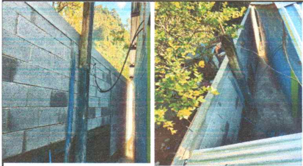
Foto 1: Reparación 18 m2 de muro perimetral de block
