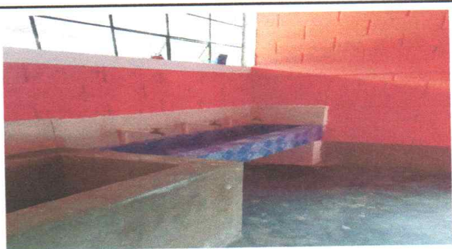
Foto9: Mejoramiento de lavamanos de concreto
