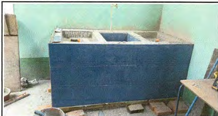
Foto 1: Instalación de azulejo en pila de cemento de dos lavaderos.
