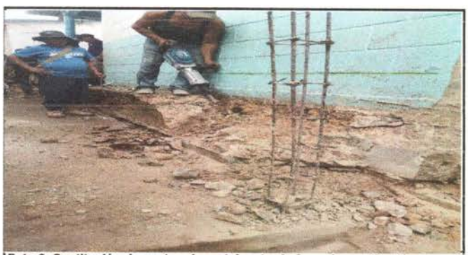
Foto 6: Sustitución de porton de metal, entrada formal y sustitución de piso de concreto
