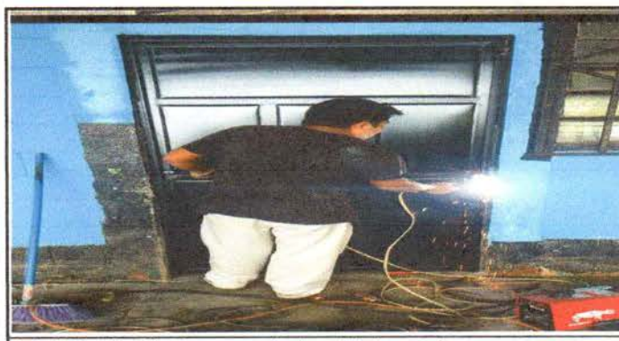
Foto 5: Sustitución de una puerta de metal de un aula.
