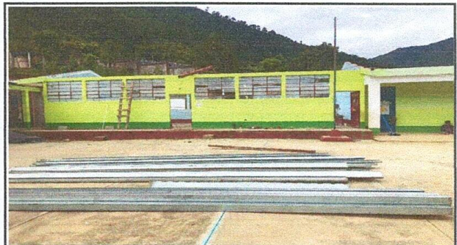
Foto 4: Colocación de lámina troquelada zinc calibre 26, capote de lámina y estructura metálica en el Módulo 1.
