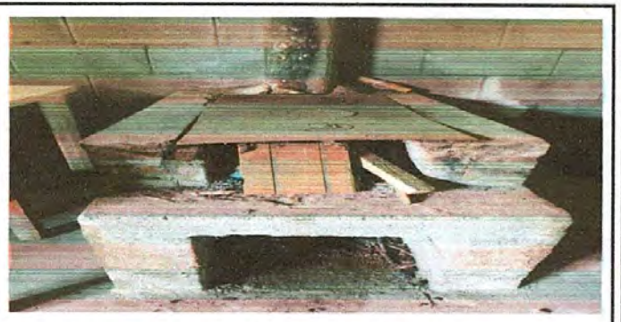
FOTO 6: Sustitución de plancha de metal de 3 hornillas
