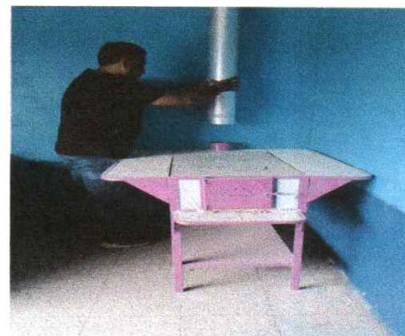
Foto 6: Instalando estufa rural
