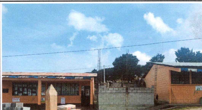
Foto 4: Sustrucción de lamina en mal estado por lamina troquelada en aula del modulo dos del Establecimiento.
