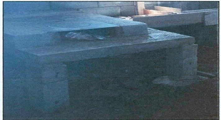
Foto 8: Sustitución de plancha de estufa de metal
