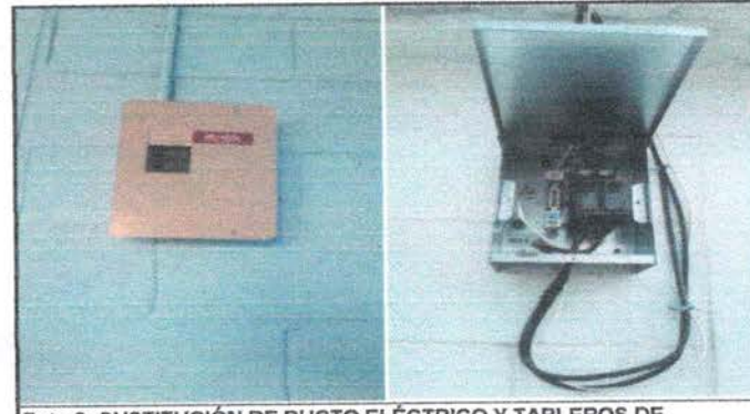
Foto 6: SUSTITUCIÓN DE DUCTO ELÉCTRICO Y TABLEROS DE FLIPONES
