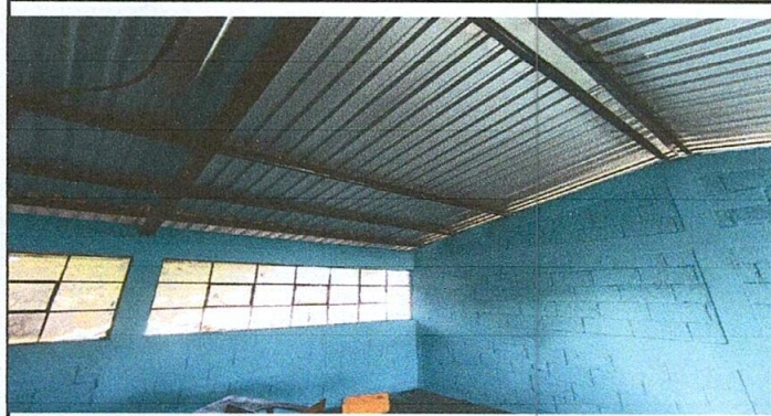
Foto1: Sustitución de Estructura de madera por metal
