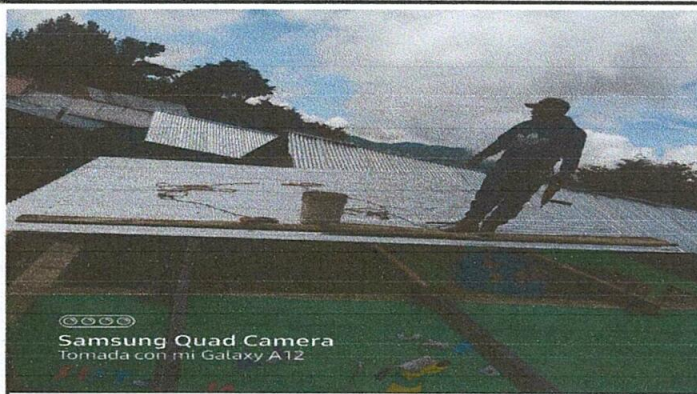
Foto 2: Sustitución de Lámina por Lámina Troquelada calibre 26
