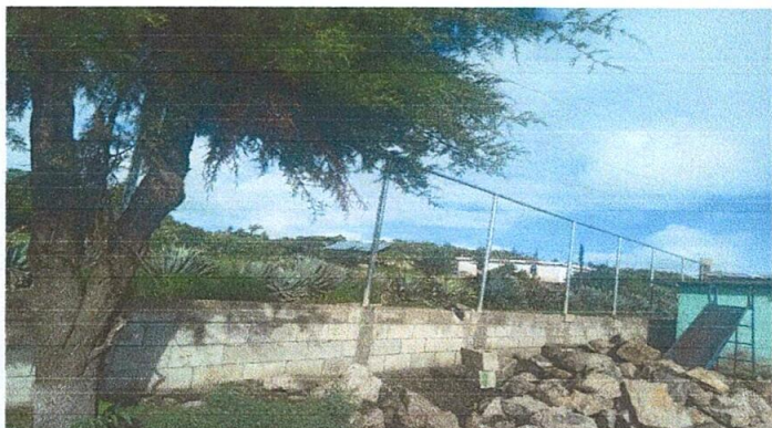
Foto 4: Reparación de muro perimetral
