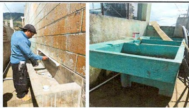
Foto 8: Red de agua potable.
