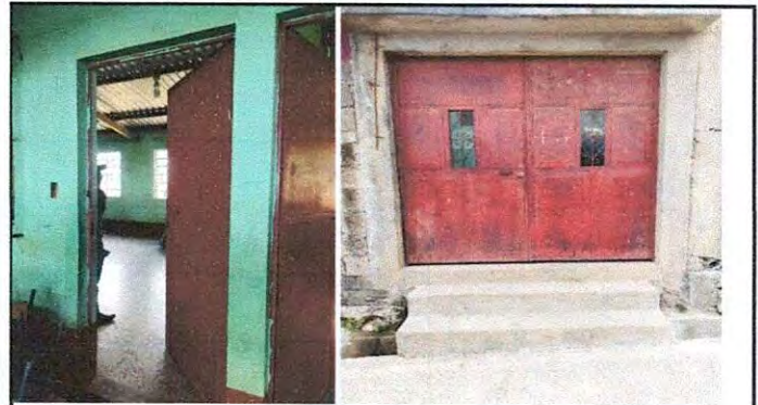
Foto 2: Aplicación de pintura externa e interna de puertas de metal.
