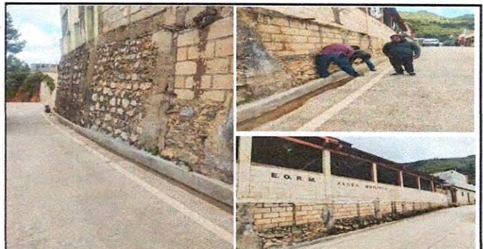
Foto 12: Reparación de muro de contención. Aplicación de sabieta en muro de contención.
