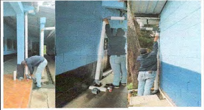
FOTO 8: Sustitución de bajada de agua pluvial por tubo PVC 4"
