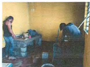
Foto19: Sustitucion de estufa rural (Completa incluye chimenea y plancha de metal)
