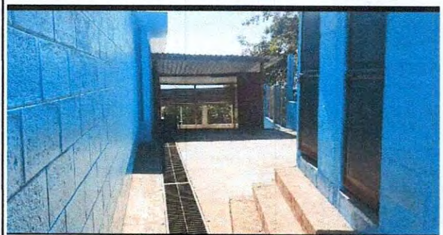
Foto 12: Parrilla para protección de cuneta
