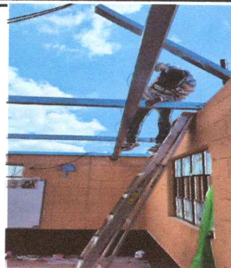
Foto 2: Sustitución de estructura de soporte de madera por metal
