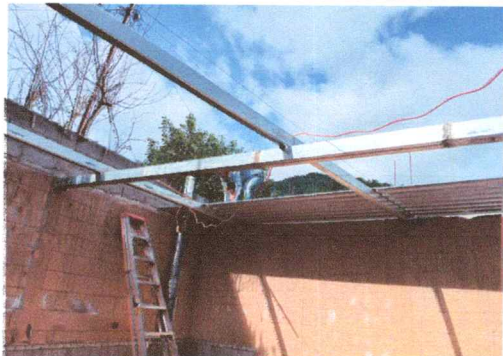
Foto1: Sustitución de lámima, por lámina troquelada aluzinc calibre 26
