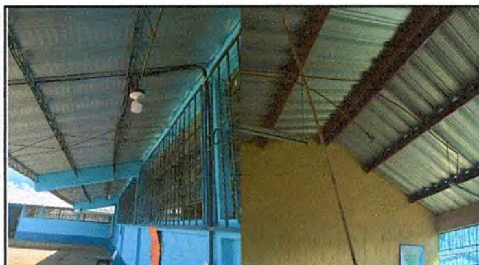
Foto 9: Sustitución de cableado eléctrico
